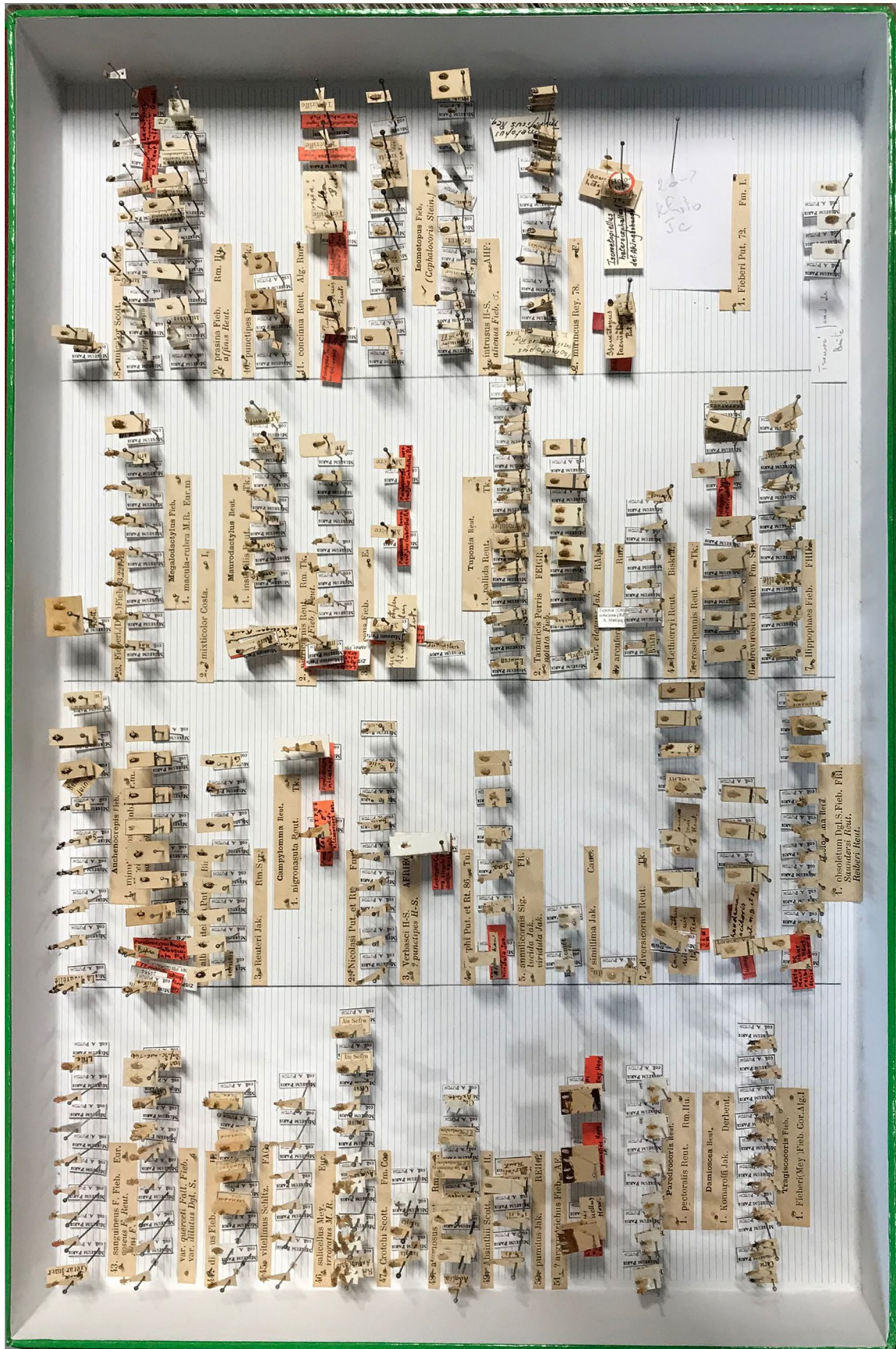
FIG. 17. — Carton 56 (Miridae) de la collection Puton, après transfert à l'identique des cartons* d'origine dans des cartons*** modernes.
