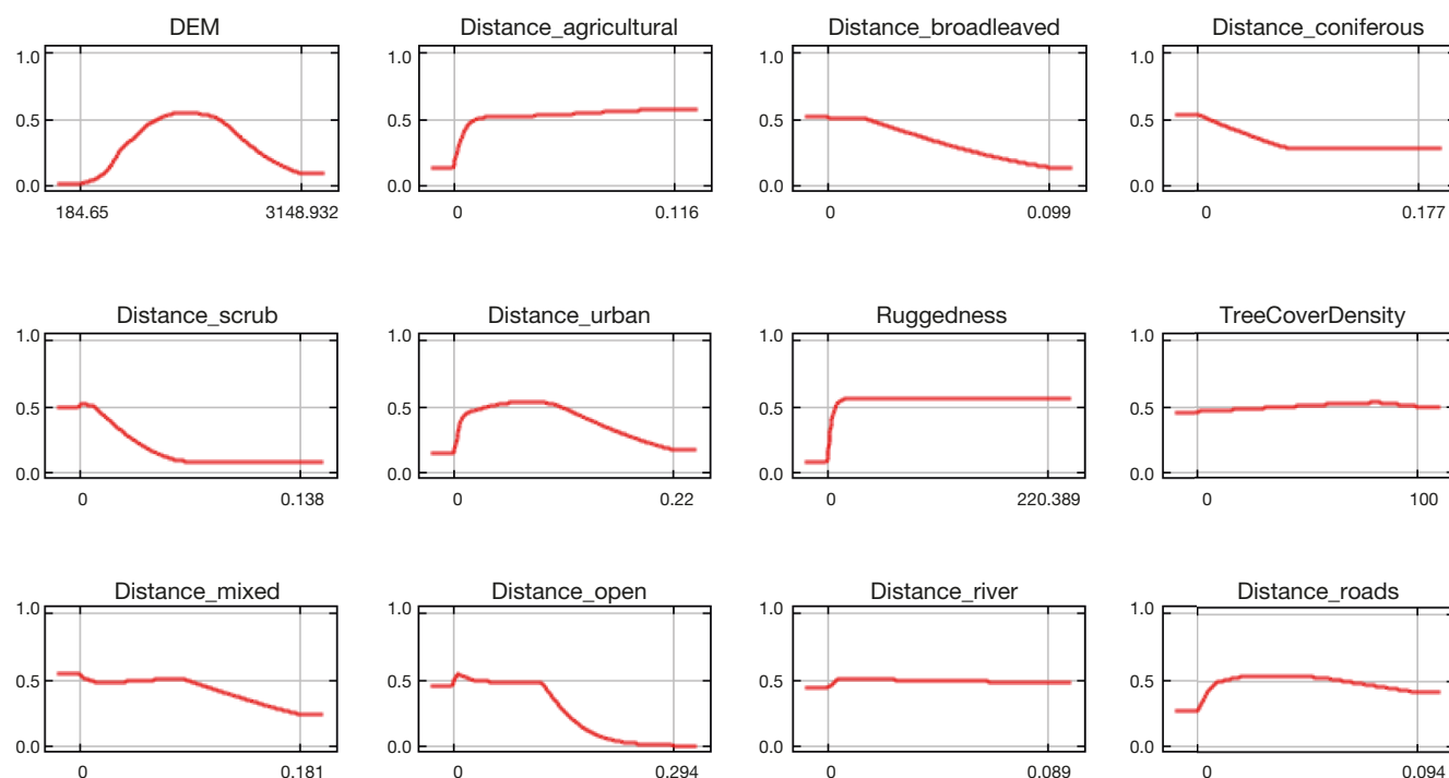
FIG. 4. — Effet des 12 variables environnementales sur l'adéquation de l'habitat de l'Ours brun Ursus arctos Linnaeus, 1758 dans les Pyrénées estimé à partir du modèle d'adéquation des habitats (MAH) implémenté sur le logiciel MaxEnt. Abréviations : DEM , altitude (selon le European Digital Elevation Model ) ; Distance_agricultural , distance à la zone agricole la plus proche ; Distance_broadleaved , distance à la forêt de feuillus la plus proche ; Distance_coniferous , distance à la forêt de conifères la plus proche ; Distance_mixed , distance à la forêt mixte la plus proche ; Distance_open , distance à la zone ouverte la plus proche ; Distance_river , distance à la rivière la plus proche ; Distance_roads , distance à la route la plus proche ; Distance_scrub , distance à la zone de broussailles la plus proche ; Distance_urban , distance à zone urbaine la plus proche ; Ruggedness , rugosité du terrain ; TreeCoverDensity , densité de couverture forestière.
