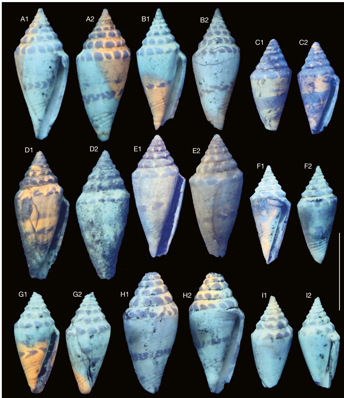
FIG. 5. — Variation of the colour pattern of Conillithes herodus n. sp. from the Tortonian of Crete (Greece): A , Paratype MNHN.F.A72587, Crete; B , Paratype MNHN.F.A72585, Crete; C , Paratype MNHN.F.A72592, Makrilia; D , Paratype MNHN.F.A72588, Crete; E , Holotype AMPG(IV) 2608, Tefeli; F , Paratype MNHN.F.A72586, Crete; G , Paratype MNHN.F.A72590, Crete; H , Paratype MNHN.F.A72589, Crete; I , Paratype MNHN.F.A72591, Crete. Scale bar: 1 cm.
