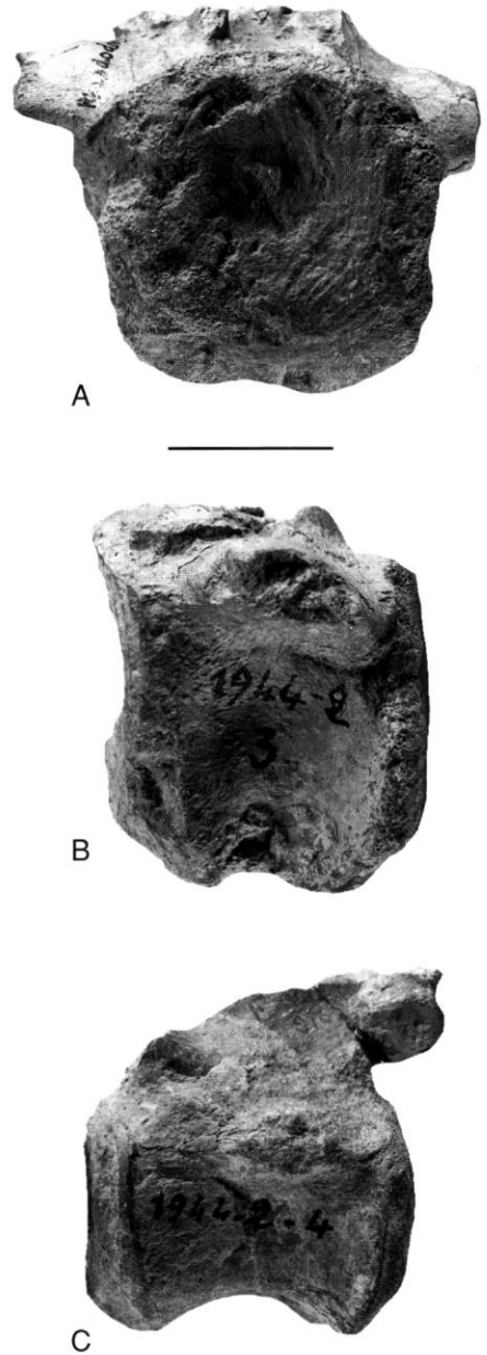
FIG. 2. — Rhabdodon sp., collection Nopcsa ; A, B, vertèbre caudale antérieure (MNHN 1944.2.3) ; A, vue postérieure ; B, vue latérale. C, vertèbre caudale moyenne, vue latérale (MNHN 1944.2.4). Échelle: 2 cm.
