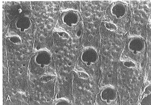
FIG. 28. — Metrarabdotos elegans Buge et Galopim de Carvalho, 1963. Saint-André-de-Bohon, est de Rougeville (Manche), niveau 26-30 m. Pliocène moyen. (R 62723 ; LP, MNHN). x 40.
