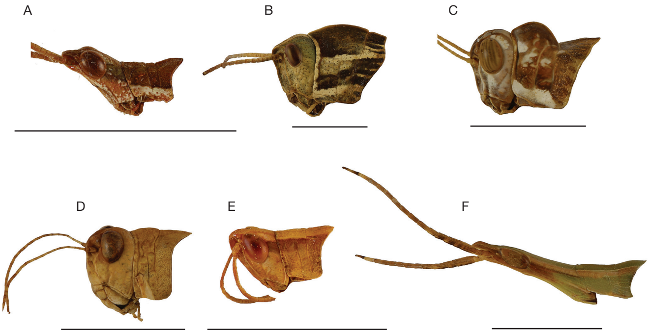
FIG. 80. — Head shape, lateral view: A , Pyrgomorpha conica (Olivier, 1791) (male); B , Pamphagus tunetanus Vosseler, 1902 (male); C , Dericorys millierei Bonnet & Finot, 1884 (female); D , Scintharista notabilis notabilis (Walker, 1870) (male); E , Duroniella lucasii Saussure, 1888 (male); F , Acrida turrita (Linnaeus, 1758) (female). Scale bars: 1 cm. Photos: H. Tlili.
