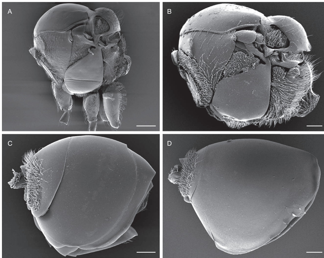
FIG. 11. — Types of mesopleura and metasomae: A , Phaenoglyphis Förster, 1869 sp.; B , C , Alloxyta Förster, 1869 sp.; D , Apocharips Fergusson, 1986 sp. Scale bars: 50 µm.
