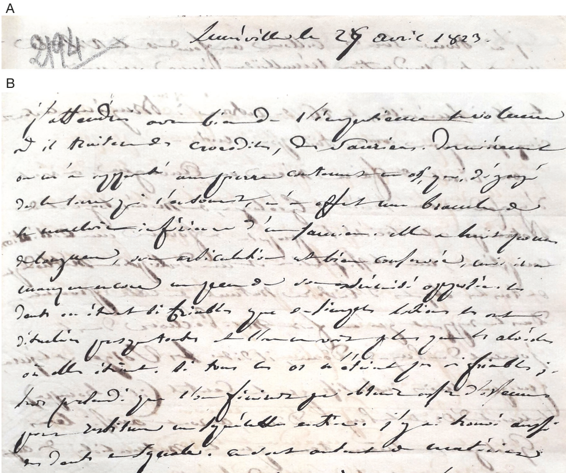
FIG. 3. — Extraits de la lettre de Charles Antoine Gaillardot à Jean-Baptiste Mugeot datée du 27 avril 1823 dans laquelle il signale la découverte d'une « branche de la mâchoire [sic] inférieure d'un saurien » (voir plus loin Fig. 7M-Q) ainsi que « des dents de squales ». © Muséum national d'Histoire naturelle, Paris (Ms 2485/2194).
